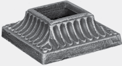
1784 ■ 11 × 11 × 3.5 cm ■ 0.55 kg 5 × 5 cm ■ اضلاع سطح مقطع
