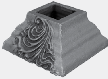
1794 ■ 14.5 × 14.5 × 7 cm ■ 1.35 kg New 5 × 5 cm ■ اضلاع سطح مقطع
