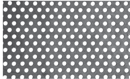
792 ■ 250 × 125 cm ■ 33 kg قطرسوراخها ■ 6 mm
