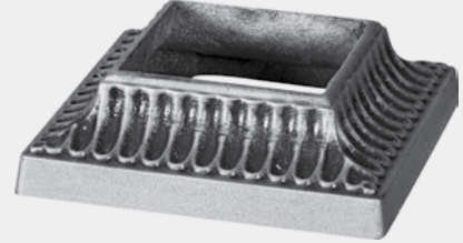
324 ■ 12.5 × 12.5 cm ■ 0.61 kg 7 × 7 cm ■ اضلاع سطح مقطع
