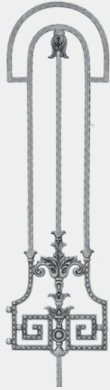
352 ■ 23 x 75 cm ■ 2.89 kg 351 ■ 23 x 90 cm ■ 3.24 kg
