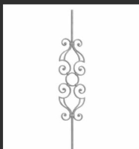
АРТИКУЛ 14-030 РАЗМЕР (1000x205x14)
