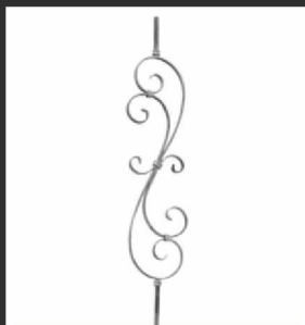
АРТИКУЛ 14-031 РАЗМЕР (1000x185x12)
